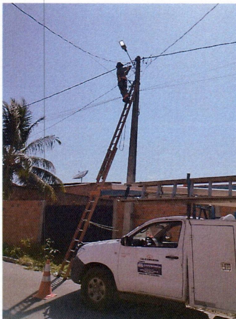
Figura 03: equipe em campo realizando substituições necessárias de Lâmpadas, cabo elétrico, conector, reator, arruela, braços com caminhonete adaptada.
