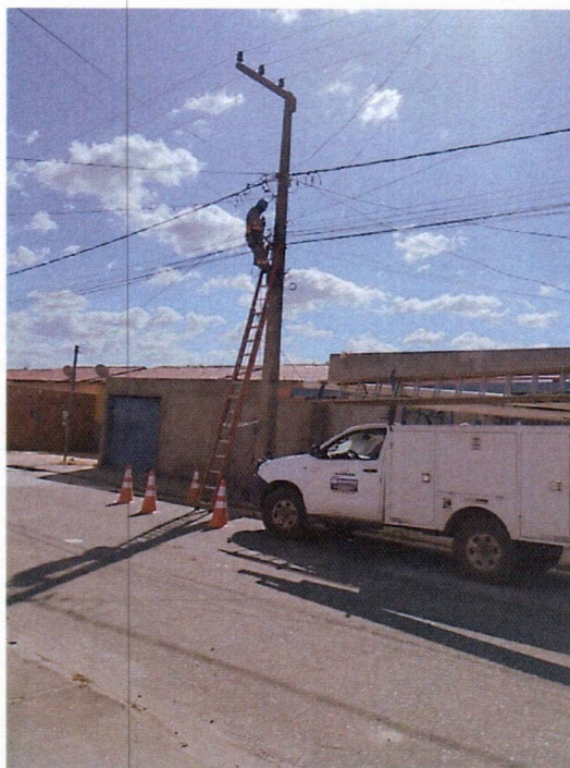
Figura 05: equipe em campo realizando substituições necessárias de Lâmpadas, cabo elétrico, conector, reator, arruela, braços com caminhonete adaptada.
