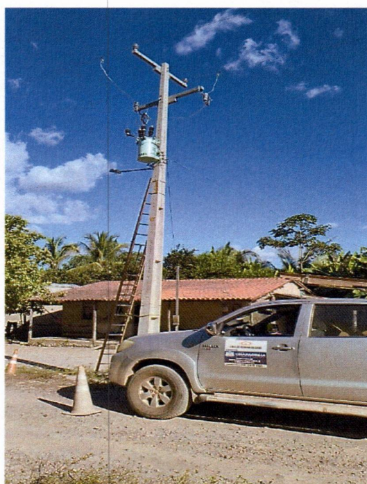
Figura 10: equipe em campo realizando substituições necessárias de Lâmpadas, cabo elétrico, conector, reator, arruela, braços com caminhonete adaptada.
