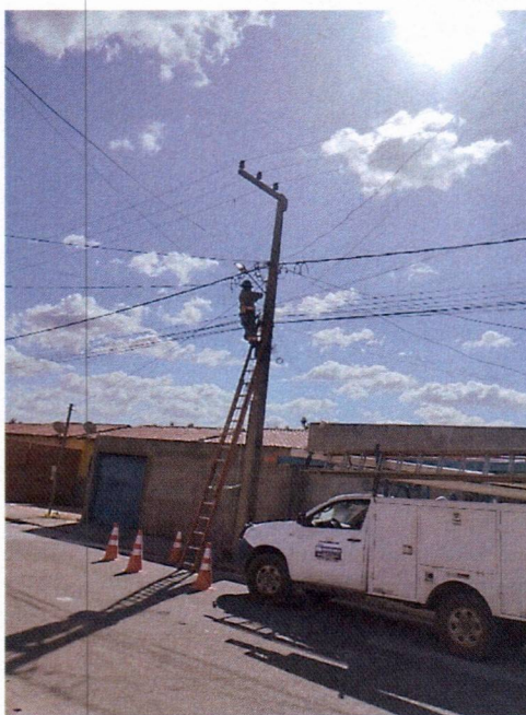
Figura 04: equipe em campo realizando substituições necessárias de Lâmpadas, cabo elétrico, conector, reator, arruela, braços com caminhonete adaptada.
