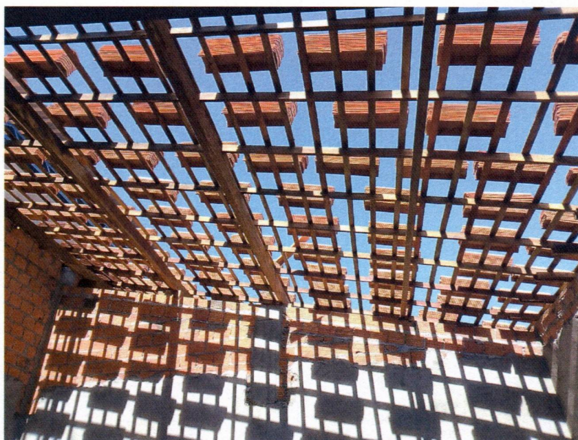
Imagem 4 – Execução da cobertura cerâmica da escola.
