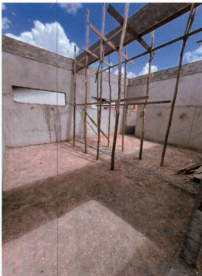
Imagem 14 – Execução de vigas, chapiscos e rebocos;
